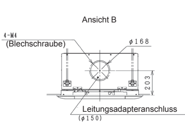
Vergrößerte Ansicht des Leitungsanschlusses (2 Seiten)
